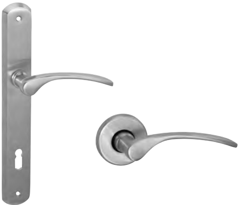
/// készleten SOFIA hosszúcímes és rozettás, matt króm F szálcsiszolt matt króm A zamak és réz M A=110 mm B=235mm C=38 mm D=50 mm
